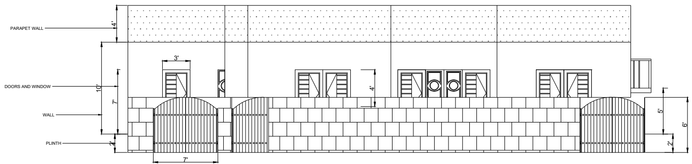
BOTTOM ELEVATION
