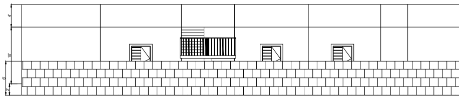
RIGHT ELEVATION
